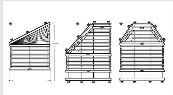
Plissee verspannt Sonderformen Modell 80339 / 80331 803341
